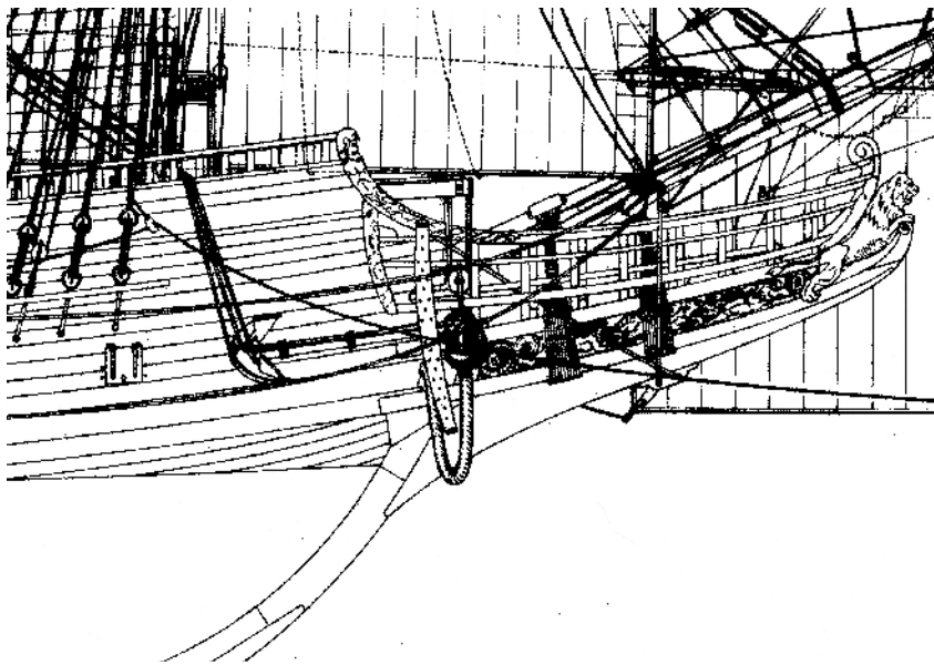
Tekening van het galjoen van een 17de-eeuws Hollands schip (de Batavia). De vloeien van het anker worden met zware touwen naar achter tegen de scheepsromp aangetrokken en vastgezet met de zogeheten penterebalk. Mogelijk heeft Guiche na zijn sprong juist die touwen kunnen vastgrijpen.
